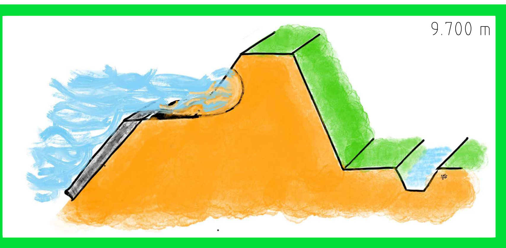
Erosie buitentalud
