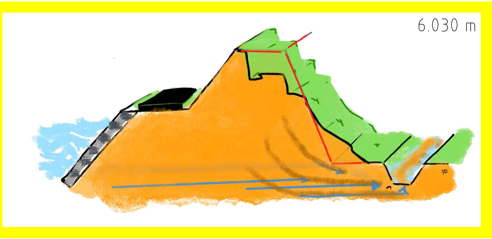
Stabiliteit steenzetting
